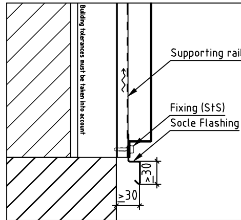
Socle
