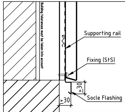
Socle
